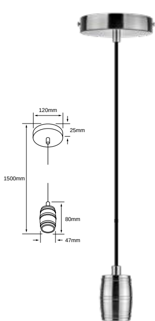
60SOCK113MVE27S ■ Satin POTENCIA: 60 W máx. LÁMPARA SUGERIDA: Filamento LED 8.5 W VOLTS: 100-240 V ~ Tipo de lámpara: Opcional (No incluida) Tipo de base: E27
