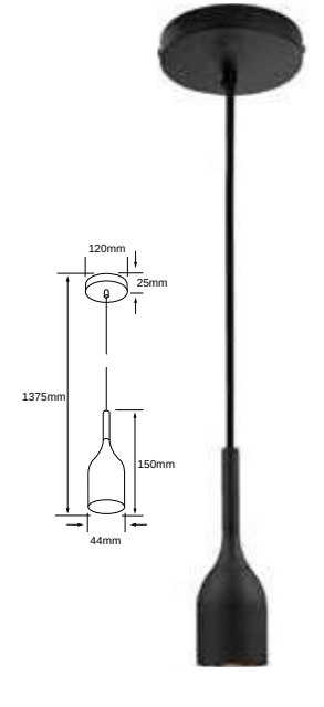
60SOCK106MVE27N ■ Negro POTENCIA: 60 W máx. LÁMPARA SUGERIDA: Filamento LED 8.5 W VOLTS: 100-240 V ~ Tipo de lámpara: Opcional (No incluida) Tipo de base: E27
